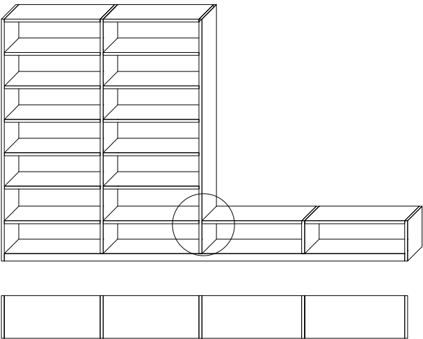
Höhenmaßwechsel ganzheitliche Komposition
