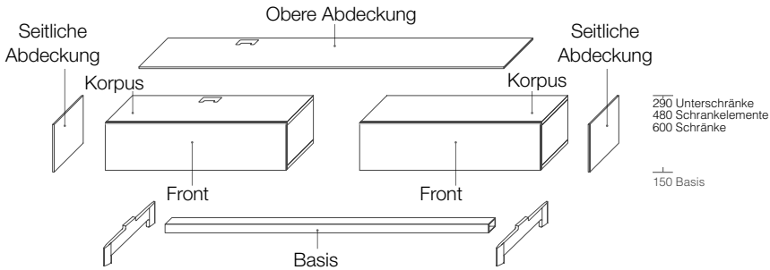
Kompositionen mit Unterschränken/Schrankelementen/Schränken mit Basis T 495
