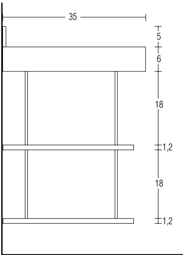
Seitenansicht Wandbefestigung
