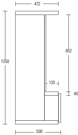
SEITLICHER ABSCHNITT
