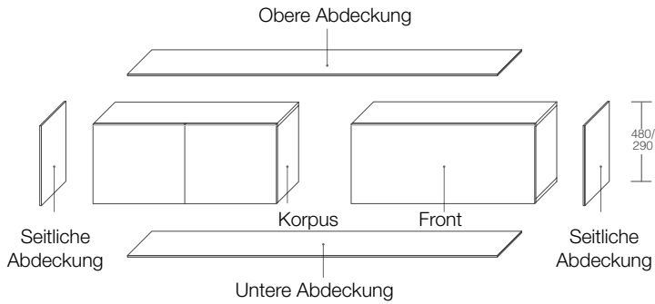
Kompositionen mit Unterschränken/Schrankelementen/Schränken mit Sockel T 495
