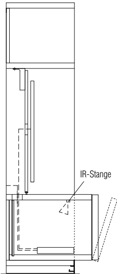
Querschnitt 3
