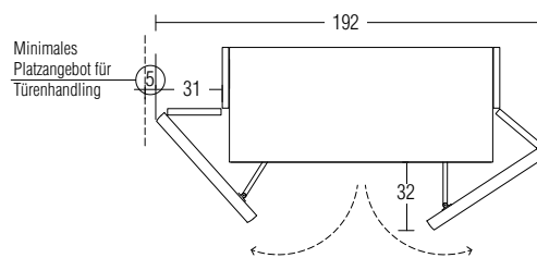
Grundriss - Abmessungen
