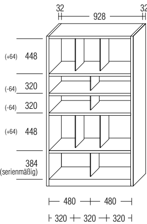
Beispiel für die Unterteilung offener Schrankelemente B 916 mit Trennwänden (Breitenpositionierung in Abständen von 160 mm)
