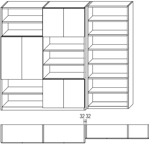
Tiefenmaßwechsel 2 Kompositionen (Beispiel 2)
