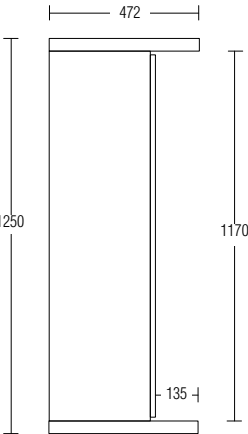
SEITLICHER ABSCHNITT
