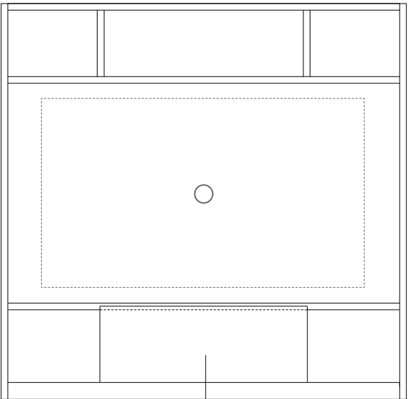
DISPLAY T 500 mit Klapptür (Querschnitt 3)
