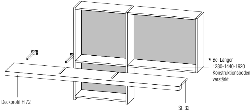
Abb. 1 - Aufbauschema
