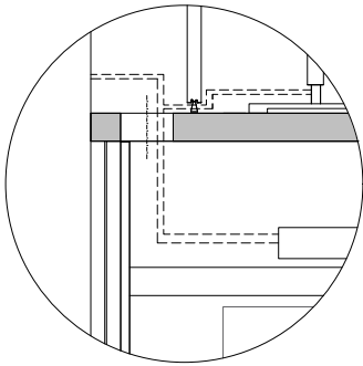
Detail A - mit aufliegendem TV
