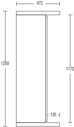
SEITLICHER ABSCHNITT
