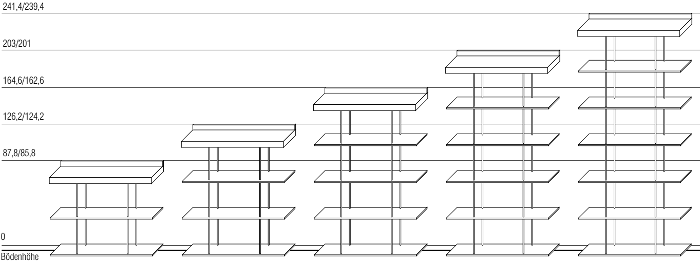
Seitenansicht Wandbefestigung
