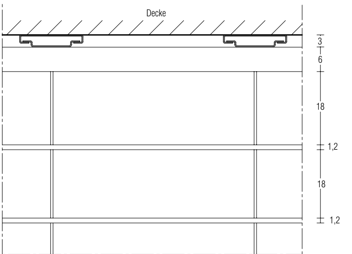
Frontansicht Deckenbefestigung
