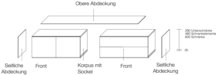
Kompositionen mit Unterschränken/Schrankelementen/Schränken mit Sockel T 495
